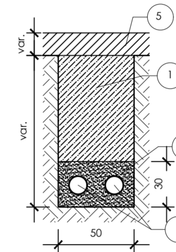
Linea su terreno (Sez A-A)
