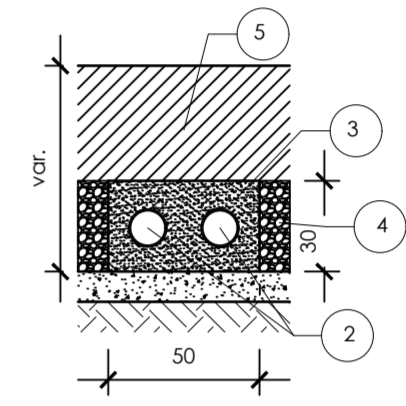
Linea su magrone esistente (Sez. B-B)
